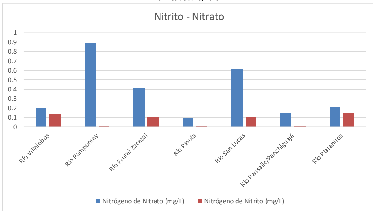
Gráfica 7: Valores de nitratos ( \text{NO}_3^- -N) y nitritos ( \text{NO}_2^- -N) de los ríos monitoreados en la Cuenca del Lago de Amatitlán durante el mes de Julio, 2025.
