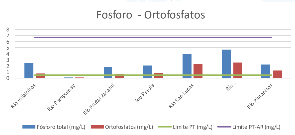
Gráfica 8: Valores de fósforo total (P) y ortofosfatos (PO 4 -P) de los ríos monitoreados en la Cuenca del Lago de Amatitlán durante el mes de Julio, 2025.
