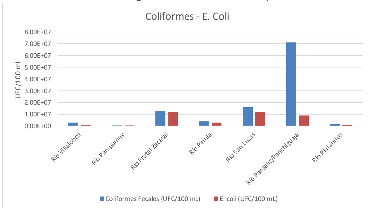
Gráfica 11: Valores de Coliformes fecales y Escherichia coli (UFC/100 ml) detectados en los ríos monitoreados en la Cuenca del Lago de Amatitlán durante el mes de Julio, 2025.
