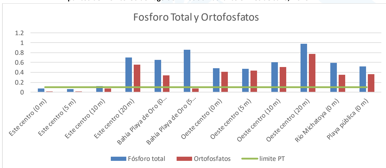
Gráfica 15: Valores de fósforo total (PT), ortofosfatos (PO 4 -P) y fósforo total disuelto (PTD) detectados en cinco puntos de monitoreo del lago de Amatitlán durante el mes de Julio, 2025.
