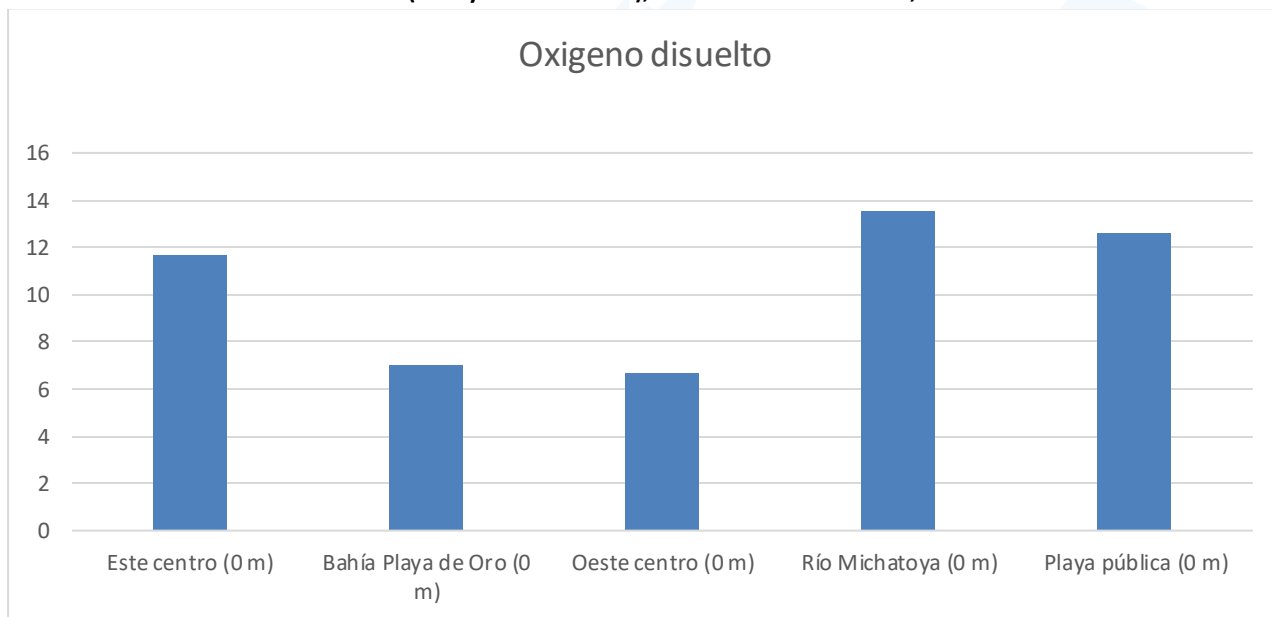
Gráfica 13: Perfil de oxígeno disuelto (mg/L) en los puntos de monitoreo que tienen la profundidad en el lago de Amatitlán (Este y Oeste Centro), durante el mes de Julio, 2025
