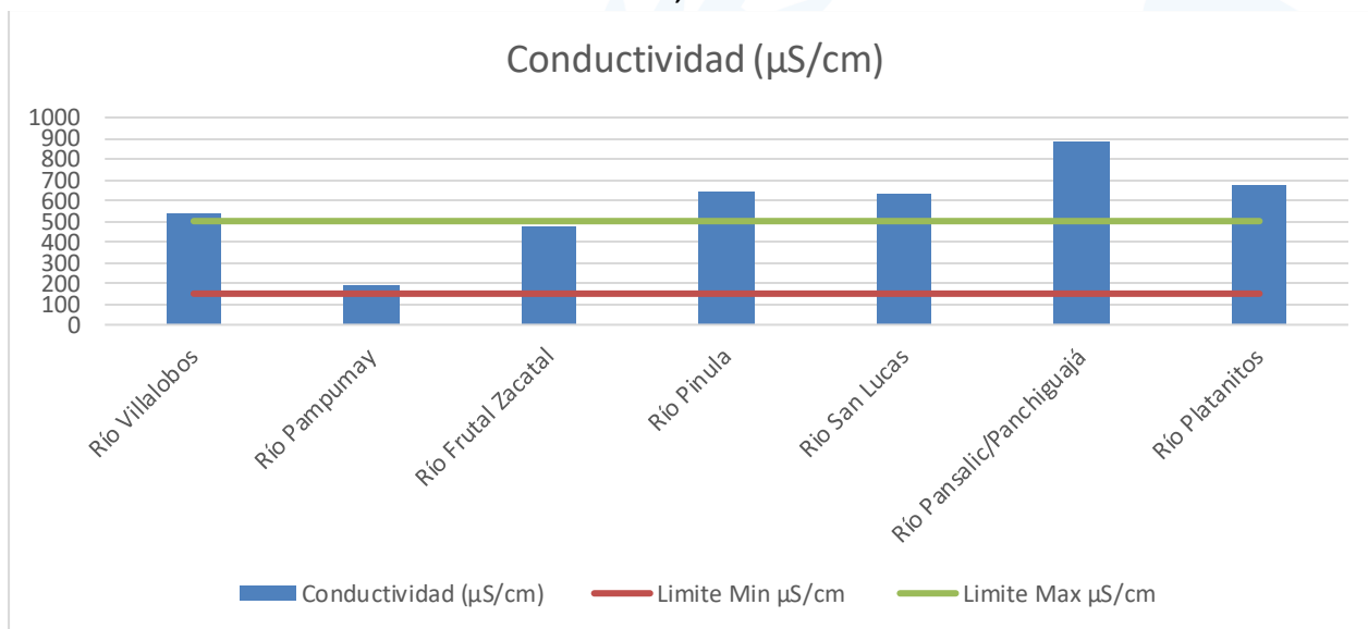
Gráfica 3: Conductividad ( \mu\text{S}/\text{cm} ) de los ríos monitoreados en la Cuenca del Lago de Amatitlán durante el mes de Julio, 2025.
