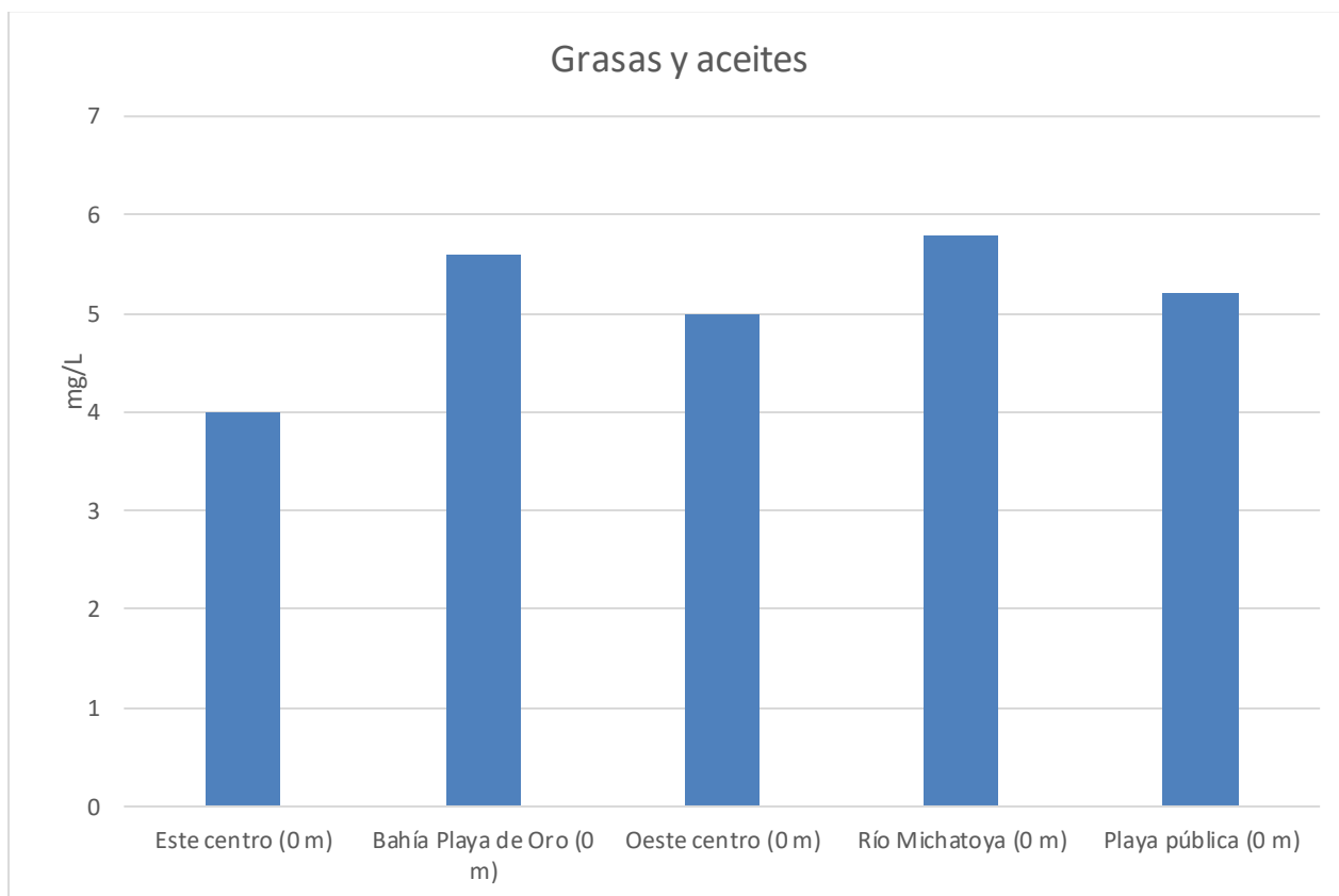
Gráfica 19: Valores de grasas y aceites (mg/L) registrados en cinco puntos de monitoreo del lago de Amatitlán durante el mes de Julio, 2025.
