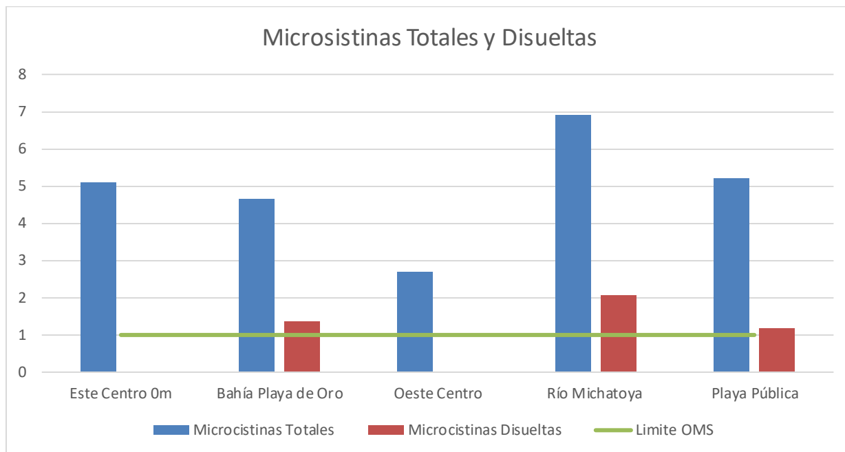
Gráfica 18: Valores de Microcistinas totales y Disueltas (mg/L) registrados en cinco puntos de monitoreo del lago de Amatitlán durante el mes de Julio, 2025.
