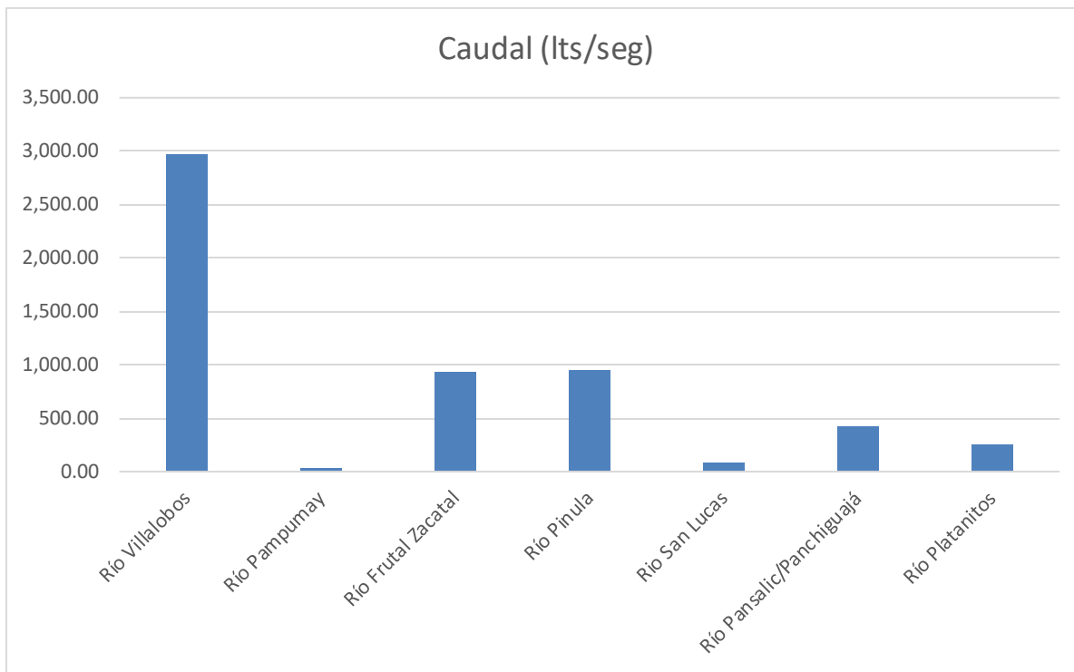
Gráfica 5: Caudal (lt/s) de los ríos monitoreados en la Cuenca del Lago de Amatitlán durante el mes de Julio, 2025.
