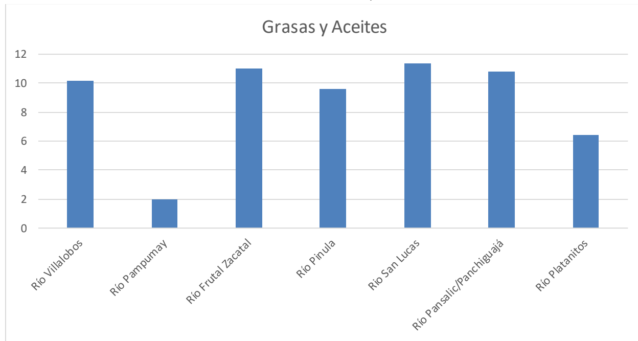
Gráfica 10: Valores de grasas y aceites (mg/L) en los ríos monitoreados de la cuenca del lago de Amatitlán durante el mes de Julio, 2025.
