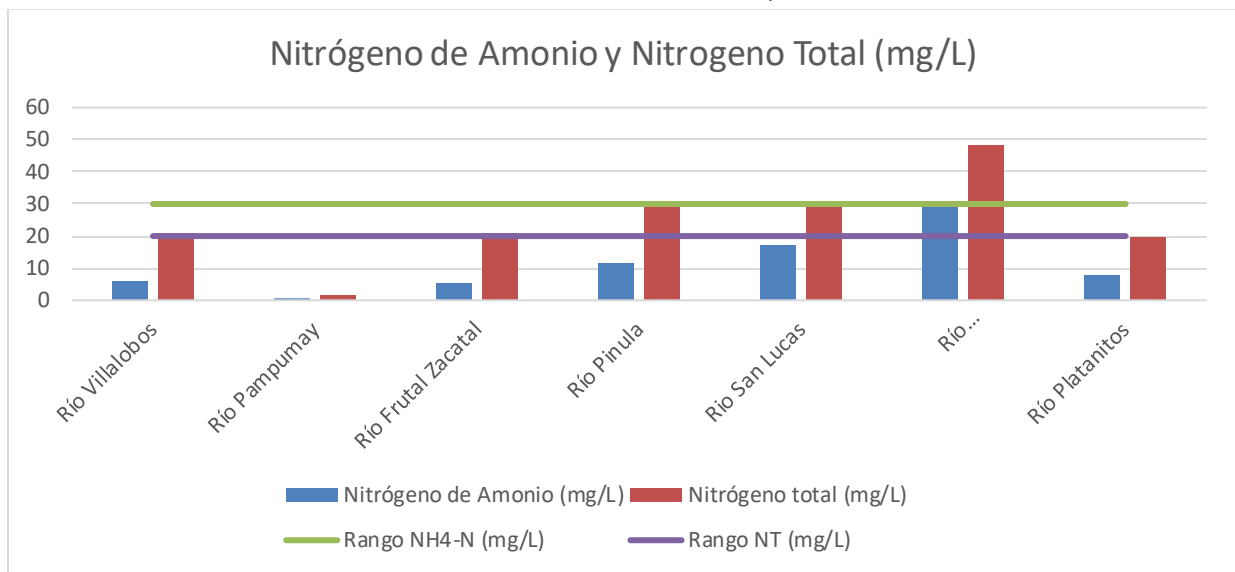
Gráfica 6: Valores de nitrógeno total (N) y amonio ( \text{NH}_3\text{-N} ) de los ríos monitoreados en la Cuenca del Lago de Amatitlán durante el mes de Julio, 2025.
