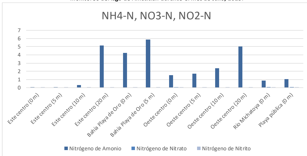
Gráfica 17: Valores de amonio ( \text{NH}_4\text{-N} ), nitratos ( \text{NO}_3\text{-N} ) y nitritos ( \text{NO}_2\text{-N} ) detectados en cinco puntos de monitoreo del lago de Amatitlán durante el mes de Julio, 2025.
