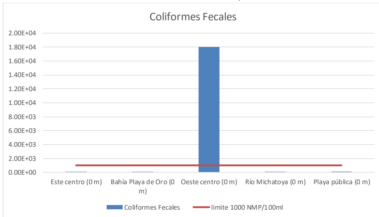
Gráfica 20: Valores de coliformes fecales (UFC/100 ml) registrados en cinco puntos de monitoreo del lago de Amatitlán durante el mes de Julio, 2025.
