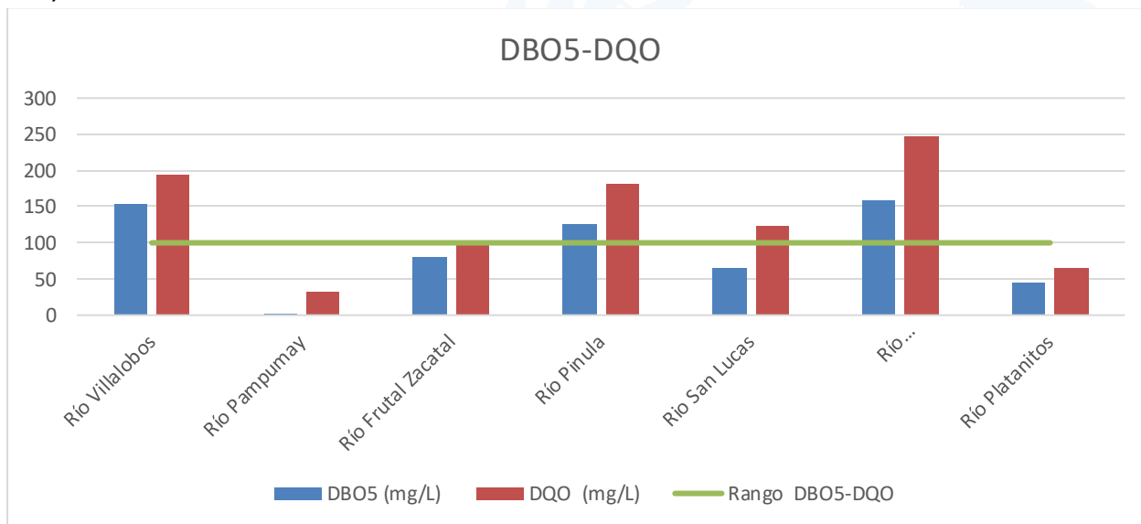
Gráfica 9: Valores de DBO 5 y DQO de los ríos muestreados de la Cuenca del lago de Amatitlán durante el mes de Julio, 2025.
