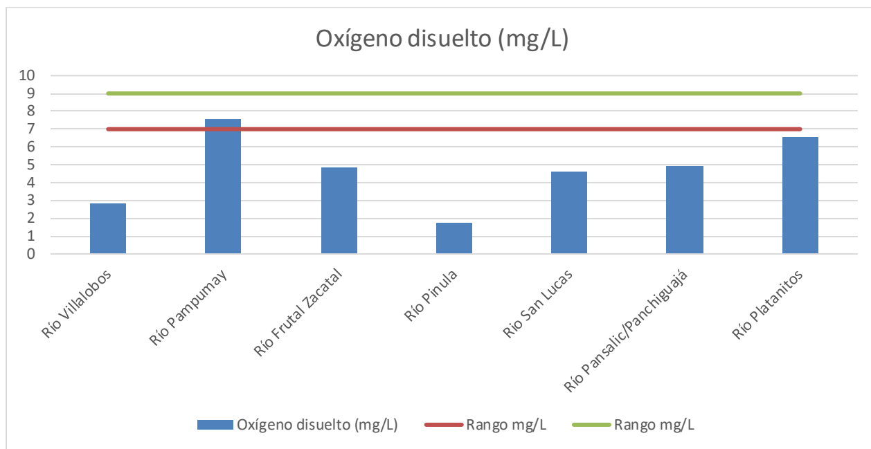
Gráfica 4: Oxígeno disuelto (mg/L) de los ríos monitoreados en la Cuenca del Lago de Amatitlán durante el mes de Julio, 2025.
