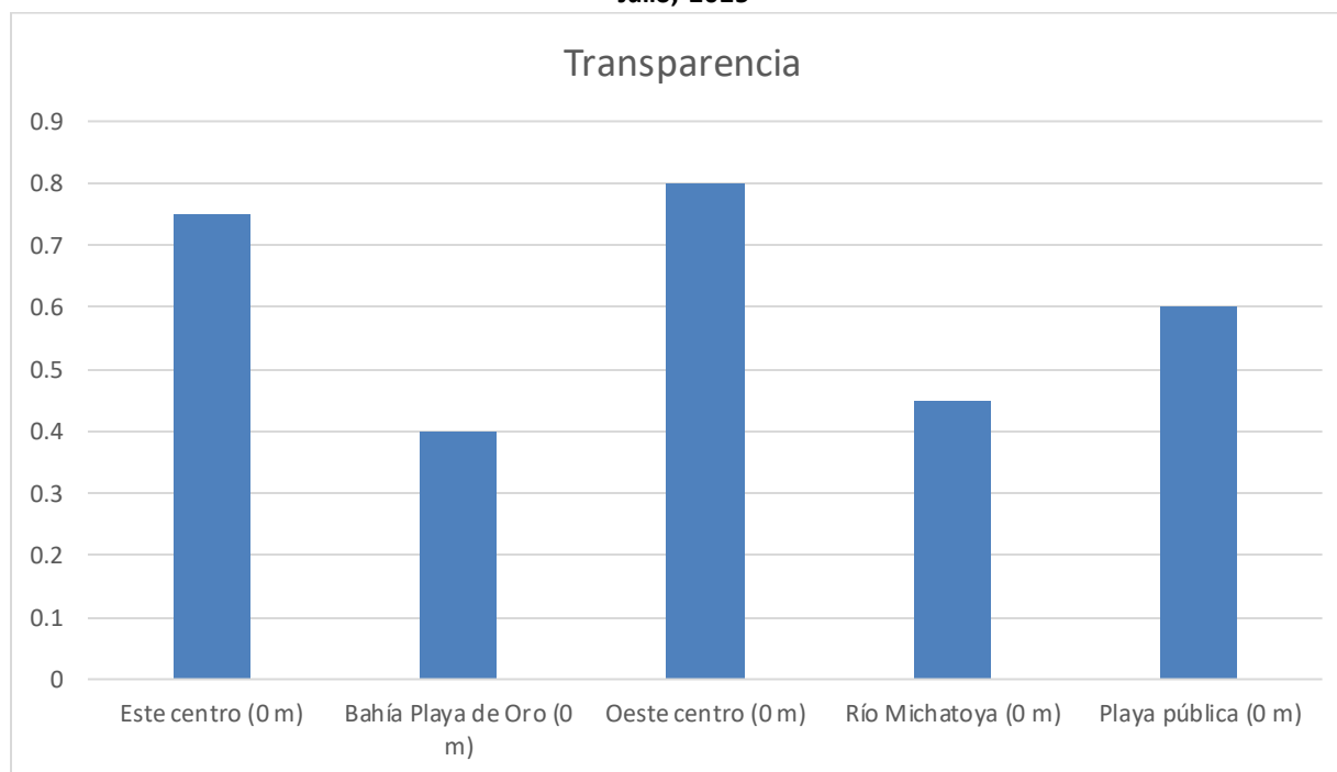
Gráfica 12: Transparencia (m) registrada en cinco puntos de monitoreo del lago de Amatitlán durante el mes de Julio, 2025
