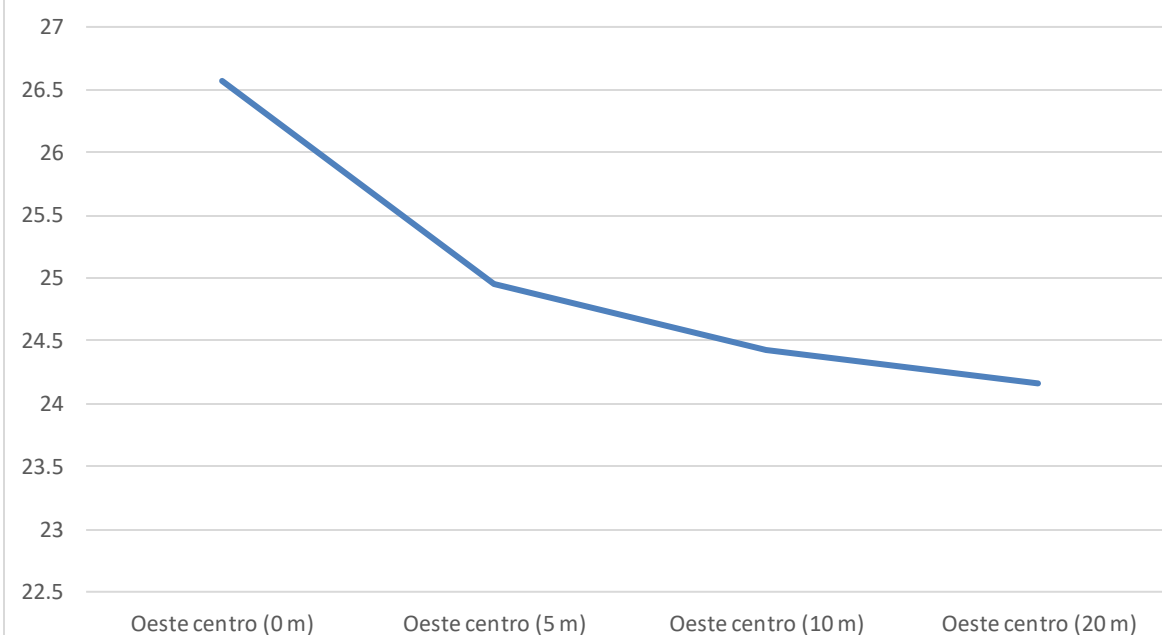
Perfil de Temperatura Oeste Centro
