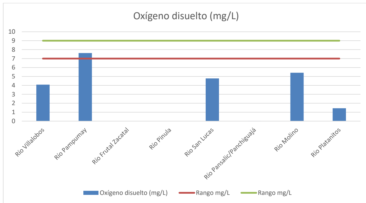
Gráfica 4: Oxígeno disuelto (mg/L) de los ríos monitoreados en la Cuenca del Lago de Amatitlán durante el mes de diciembre, 2025.
