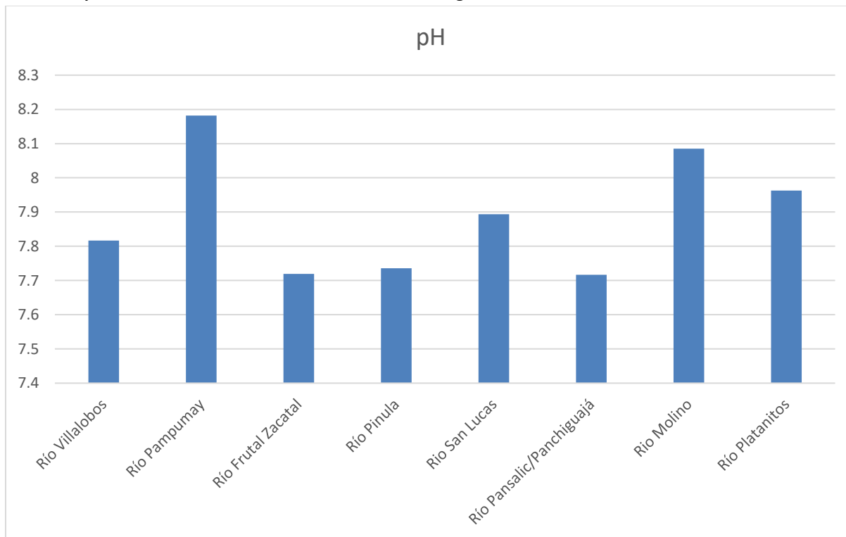
Gráfica 1: pH de los ríos monitoreados en la Cuenca del Lago de Amatitlán durante el mes de diciembre, 2025.
