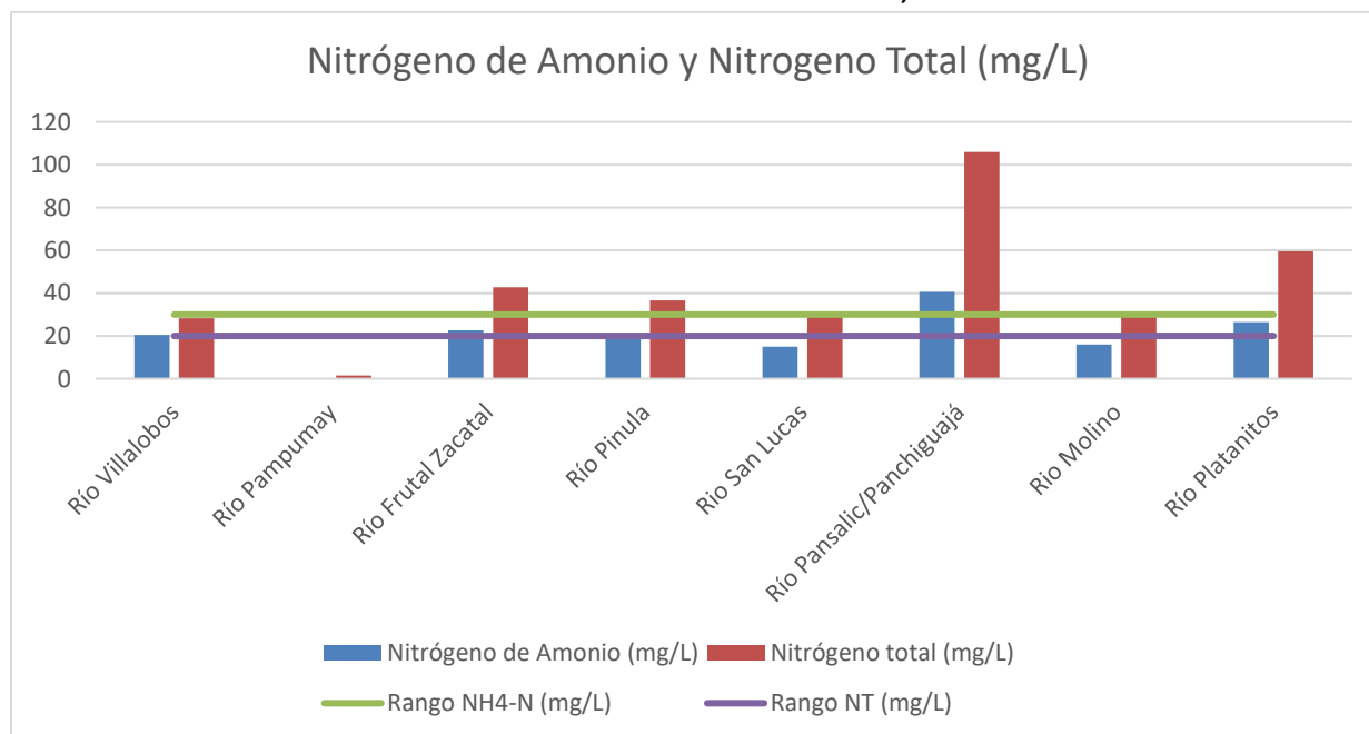
Gráfica 6: Valores de nitrógeno total (N) y amonio ( \text{NH}_3\text{-N} ) de los ríos monitoreados en la Cuenca del Lago de Amatitlán durante el mes de diciembre, 2025.
