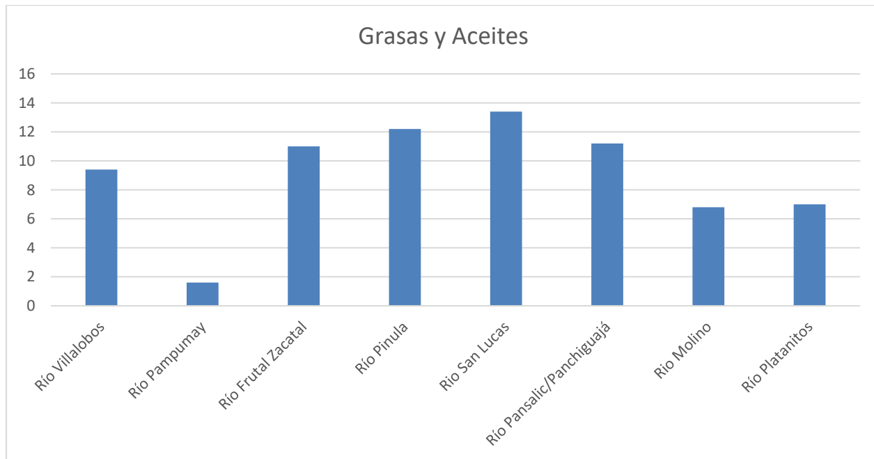
Gráfica 10: Valores de grasas y aceites (mg/L) en los ríos monitoreados de la cuenca del lago de Amatitlán durante el mes de diciembre, 2025.
