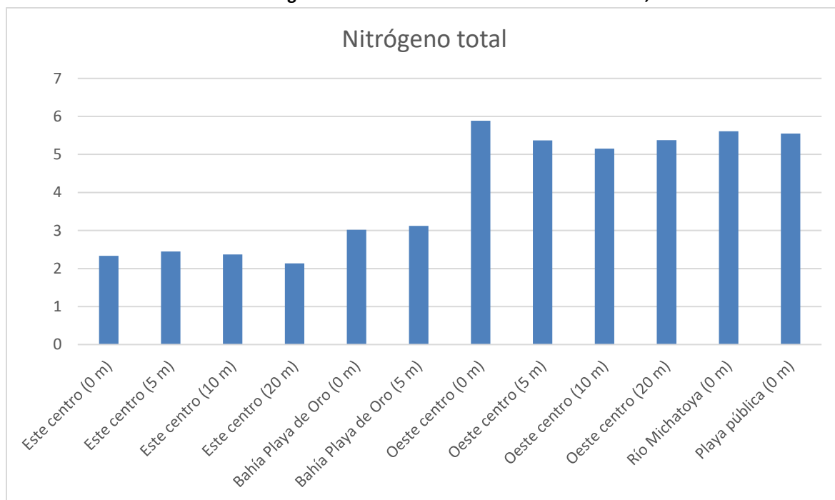
Gráfica 16: Valores de nitrógeno total (NT) y nitrógeno total disuelto (NTD) detectados en cinco puntos de monitoreo del lago de Amatitlán durante el mes de diciembre, 2025.
