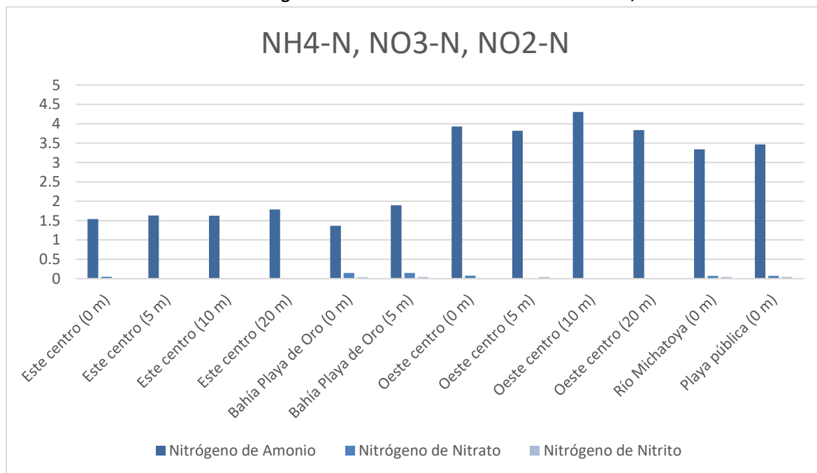
Gráfica 17: Valores de amonio (NH 4 -N), nitratos (NO 3 -N) y nitritos (NO 2 -N) detectados en cinco puntos de monitoreo del lago de Amatitlán durante el mes de diciembre, 2025.
