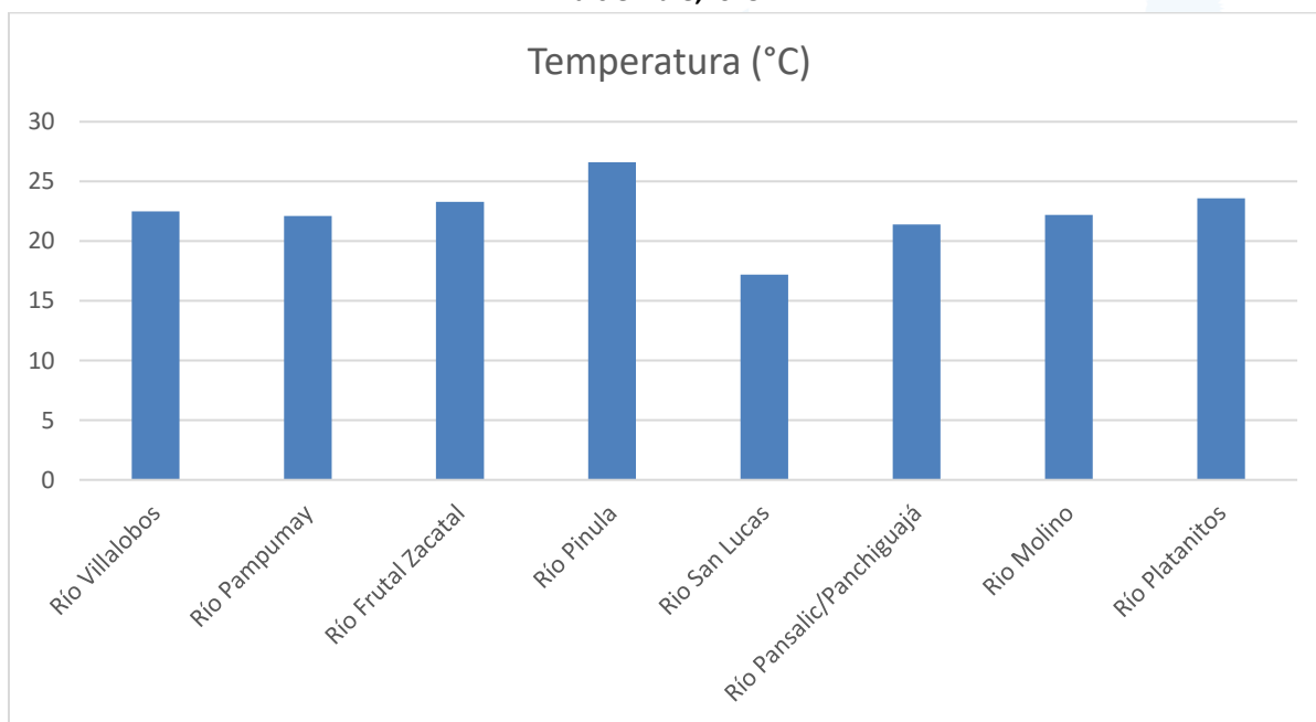
Gráfica 2: Temperatura (°C) de los ríos monitoreados en la Cuenca del Lago de Amatitlán durante el mes de diciembre, 2025.
