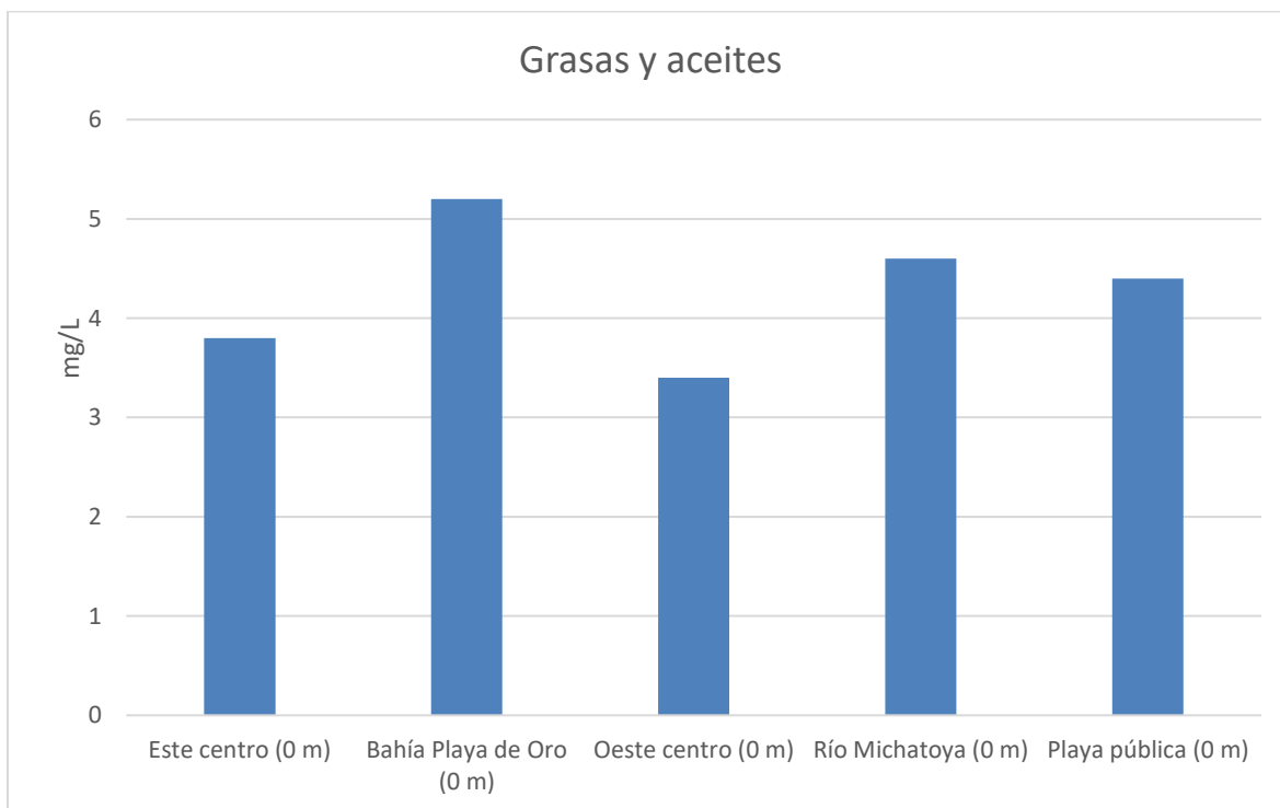
Gráfica 19: Valores de grasas y aceites (mg/L) registrados en cinco puntos de monitoreo del lago de Amatitlán durante el mes de diciembre, 2025.
