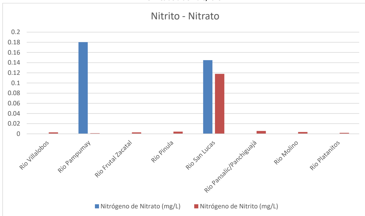
Gráfica 7: Valores de nitratos ( \text{NO}_3^- -N) y nitritos ( \text{NO}_2^- -N) de los ríos monitoreados en la Cuenca del Lago de Amatitlán durante el mes de diciembre, 2025.
