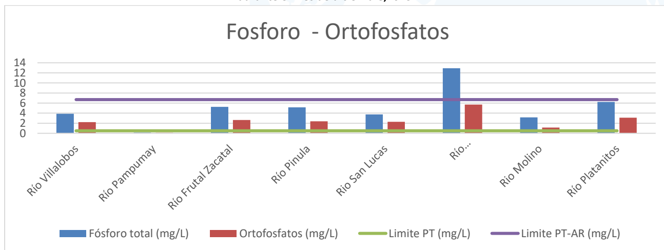
Gráfica 8: Valores de fósforo total (P) y ortofosfatos (PO 4 -P) de los ríos monitoreados en la Cuenca del Lago de Amatitlán durante el mes de diciembre, 2025.
