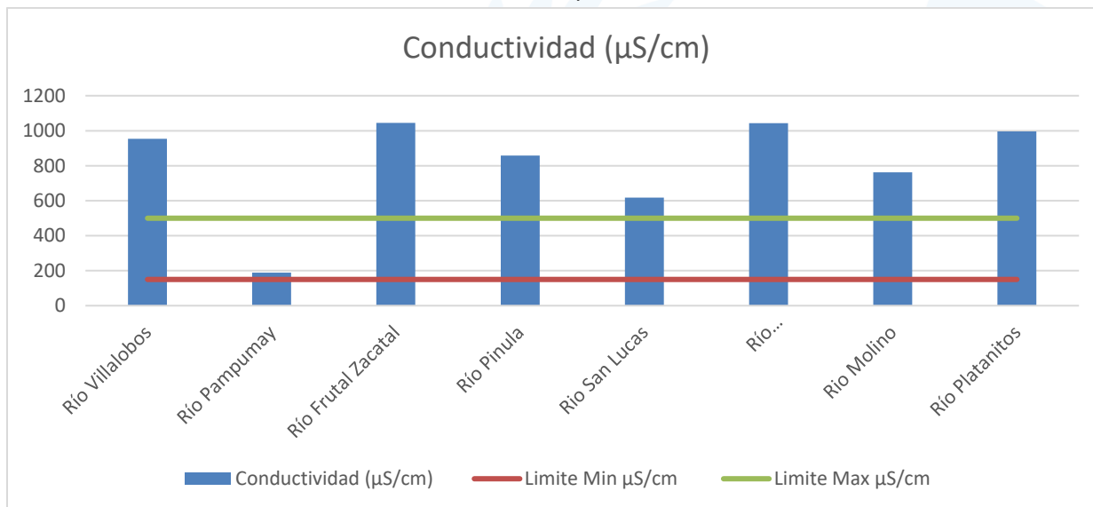
Gráfica 3: Conductividad ( \mu\text{S}/\text{cm} ) de los ríos monitoreados en la Cuenca del Lago de Amatitlán durante el mes de diciembre, 2025.
