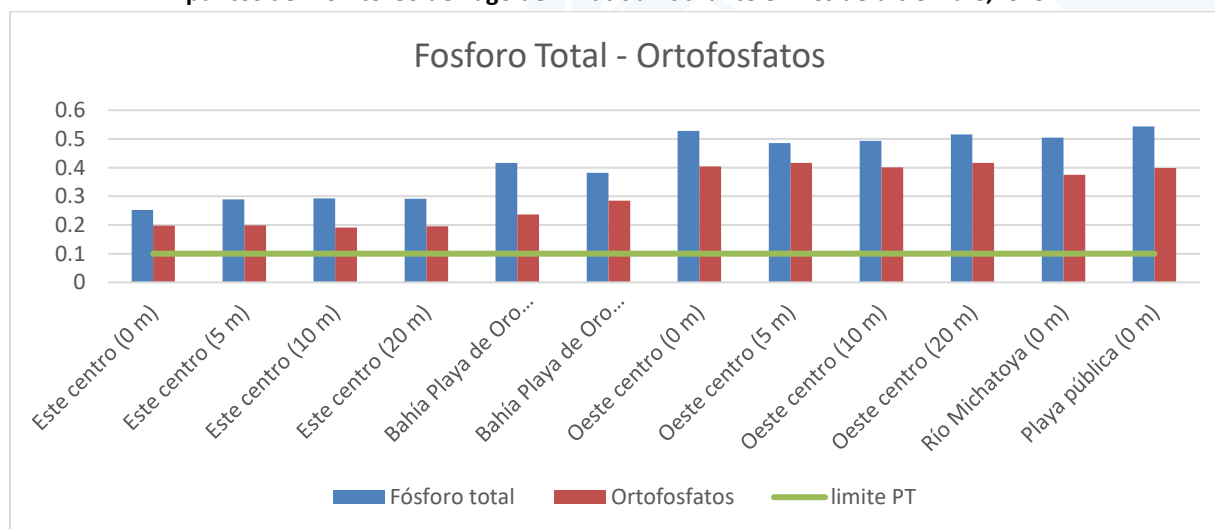
Gráfica 15: Valores de fósforo total (PT), ortofosfatos (PO4-P) y fósforo total disuelto (PTD) detectados en cinco puntos de monitoreo del lago de Amatitlán durante el mes de diciembre, 2025.
