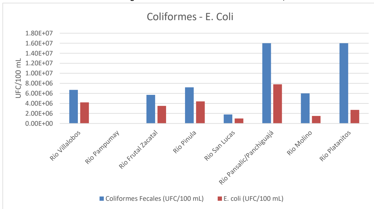
Gráfica 11: Valores de Coliformes fecales y Escherichiacoli (UFC/100 ml) detectados en los ríos monitoreados en la Cuenca del Lago de Amatitlán durante el mes de diciembre, 2025.
