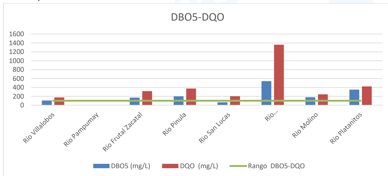
Gráfica 9: Valores de DBO 5 y DQO de los ríos muestreados de la Cuenca del lago de Amatitlán durante el mes de diciembre, 2025.
