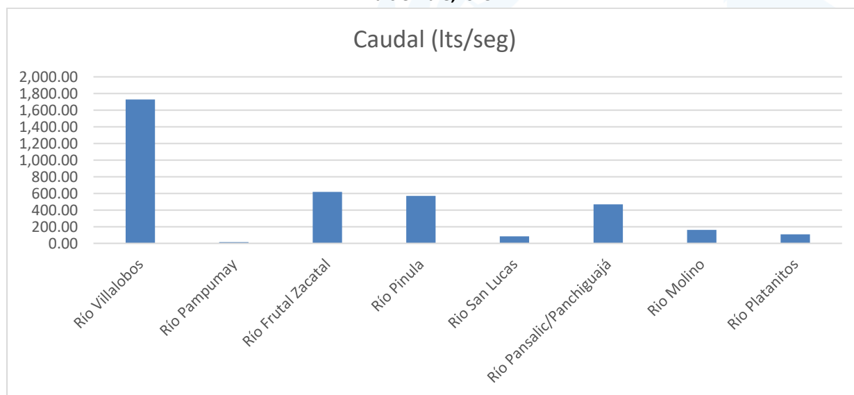
Gráfica 5: Caudal (lt/s) de los ríos monitoreados en la Cuenca del Lago de Amatitlán durante el mes de diciembre, 2025.
